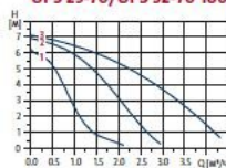
UPS 25-70/UPS 32-70 180
